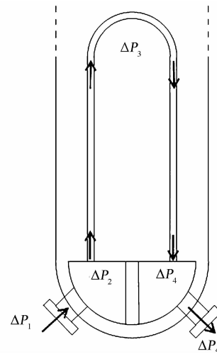
图1 一次侧流体流动示意图
